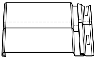
DÉTAIL DE CHEVAUCHEMENT
